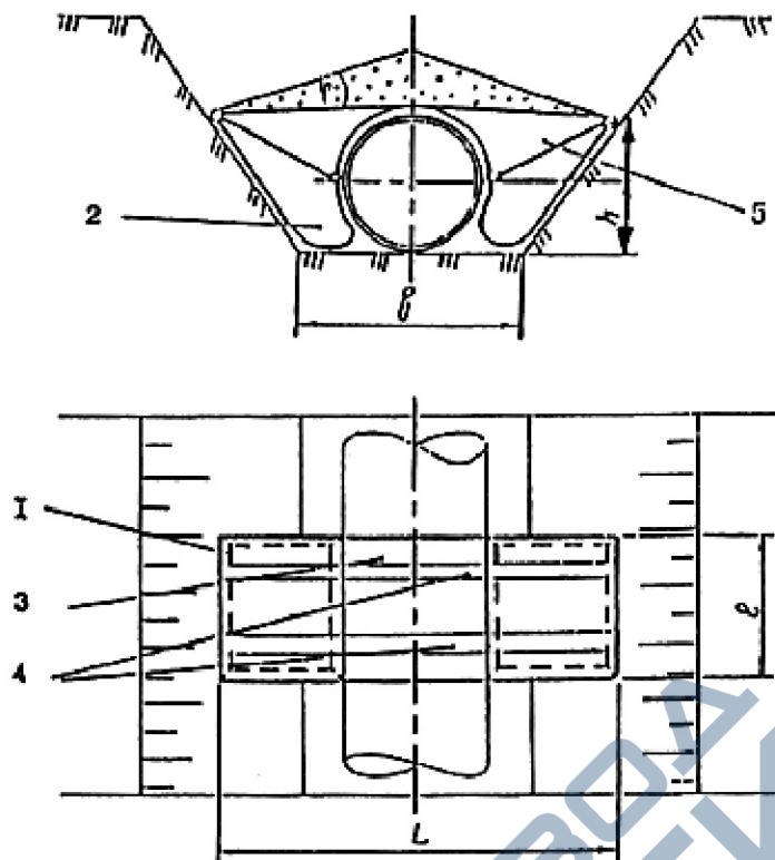
Рис. 3. Схема конструкции полимерно-контейнерного балластирующего устройства:
