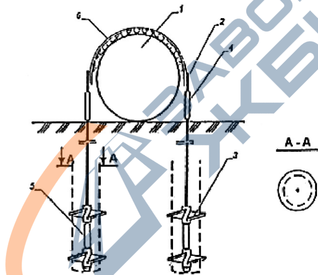
Рис. 13. Винтовое вмораживаемое анкерное устройство ВАУ-В:
