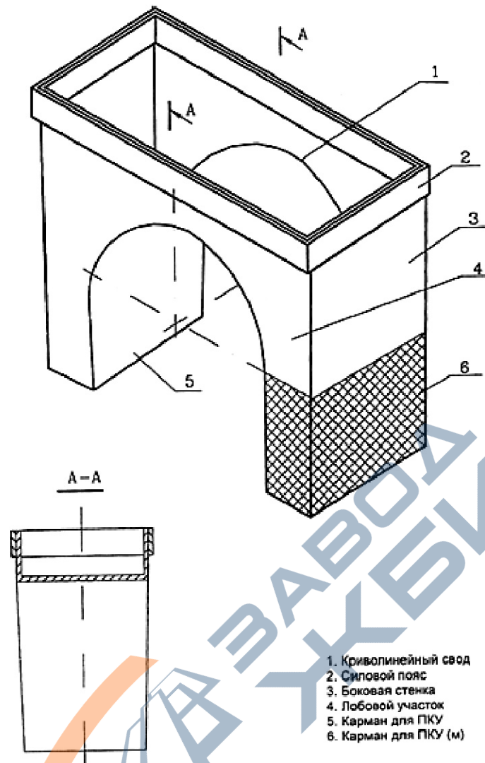
Рис. 18. Полимерконтейнер ПКУ
