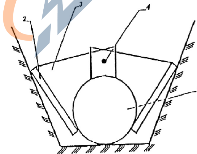
Рис. 9. Железобетонный утяжелитель типа УБТ:
