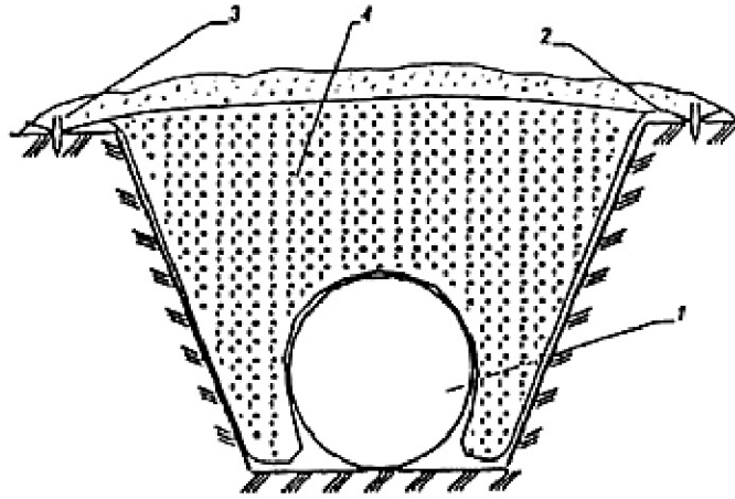
Рис. 14. Способ балластирования газопроводов минеральным грунтом засыпки с использованием полотнищ из НСМ (для песчаных грунтов) - схема 1:
